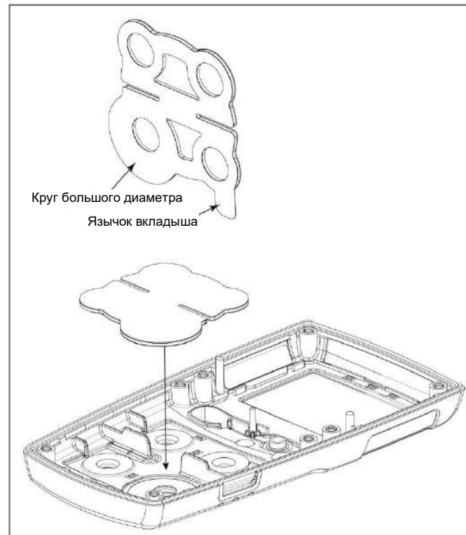
Рис. 10 Язычок вкладыша
