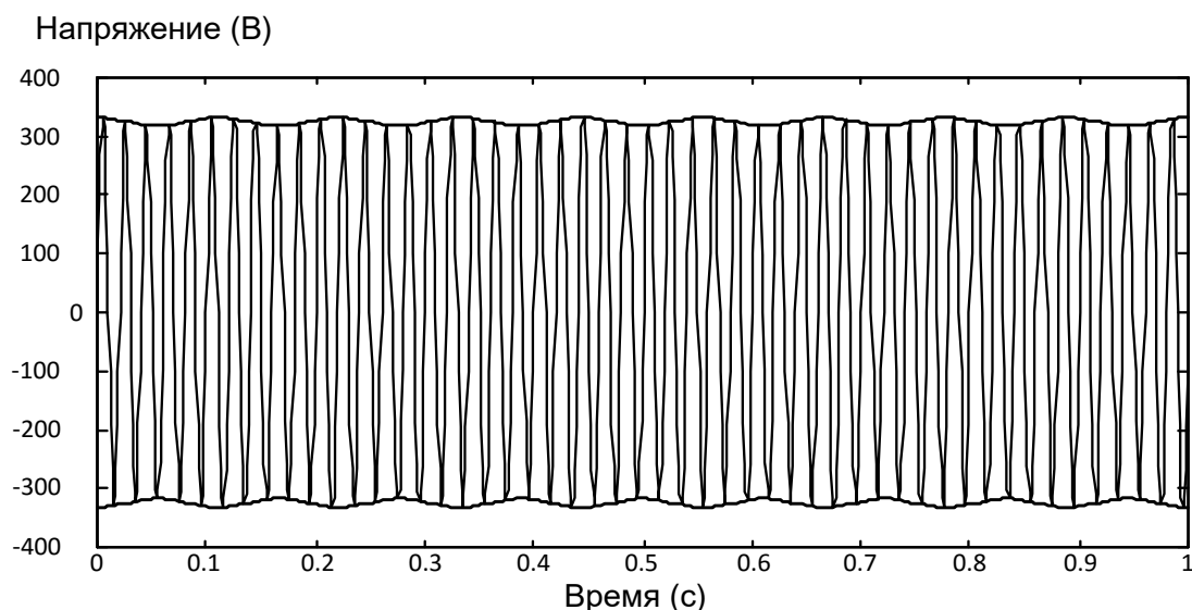
Рисунок 5.8: Колебания напряжения
