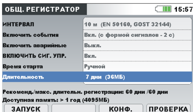
Рисунок 5.25: Предварительно определенная конфигурация регистратора в соответствии со стандартом EN50160.
