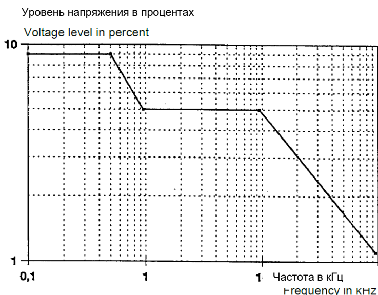
Рисунок 5.24: Предельные уровни сигнальных напряжений, передаваемых по электрическим сетям, согласно стандарту EN50160
