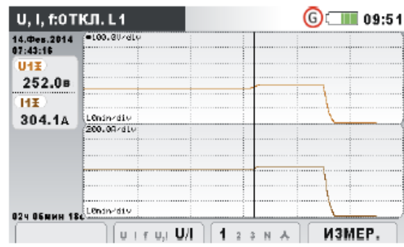
Рисунок 3.19: Отклонения напряжения и тока (двухмодовый режим)
