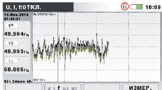
Рисунок 3.21: Отклонения частоты
