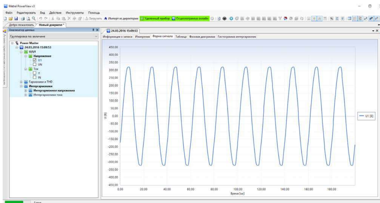
Рисунок 4.35: Окно осциллограммы в реальном времени при удаленном подключении
