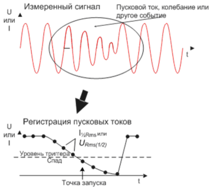
Рисунок 5.25: Триггерные сигналы по уровню
