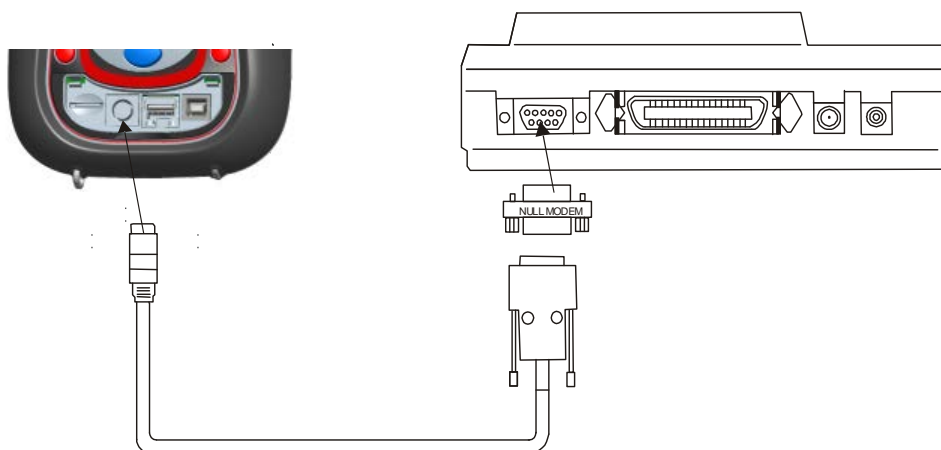
Рисунок 4.24: Подключение прибора к принтеру DPU 414
