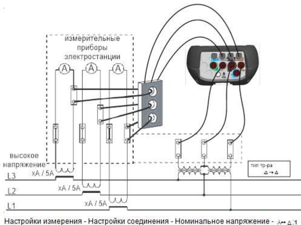
Рисунок 4.13: Подключение прибора к существующим трансформаторам тока в системе среднего напряжения (Аарон/ открытый треугольник)
