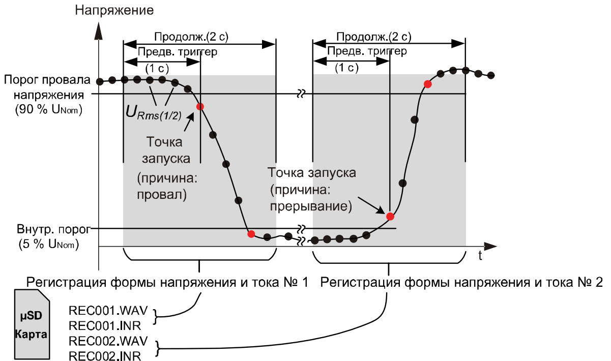
Рисунок 5.21: Сигнал триггера по событию напряжения
