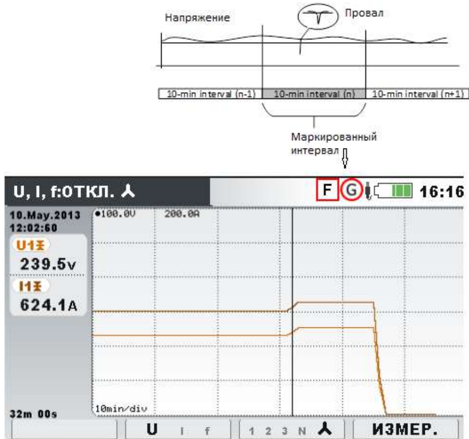
Рисунок 5.19: Маркировка данных указывает, что объединенное значение может быть недостоверным
