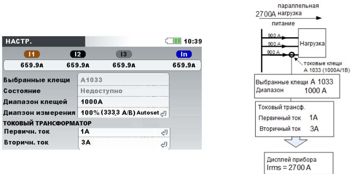
Рисунок 4.18: Параллельное питание большой нагрузки
