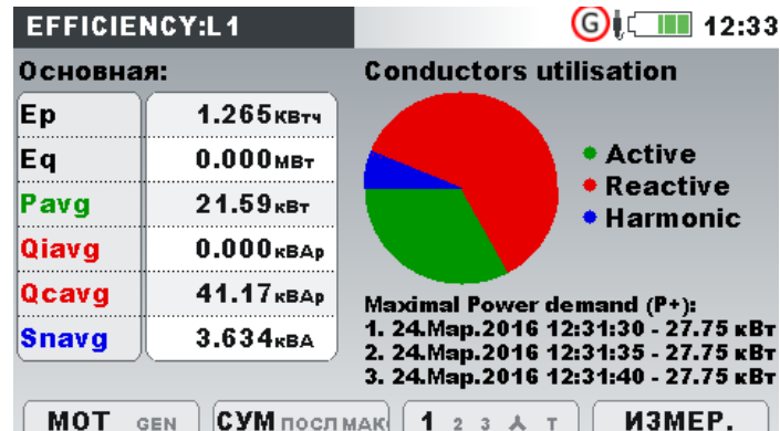
Рисунок 3.3: Экран энергоэффективности
