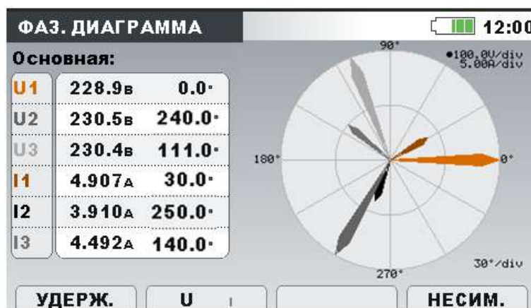
Рисунок 3.1: Экран фазовой диаграммы
