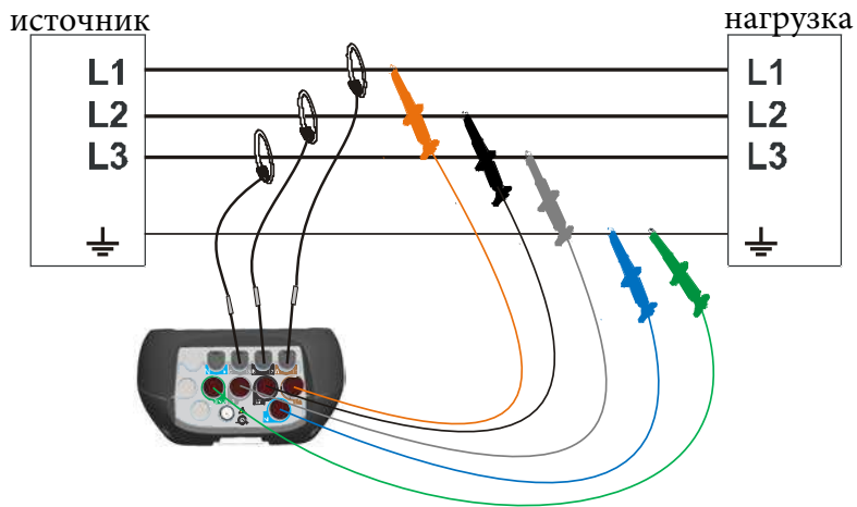
Рисунок 4.5: 3-фазная 3-проводная система
