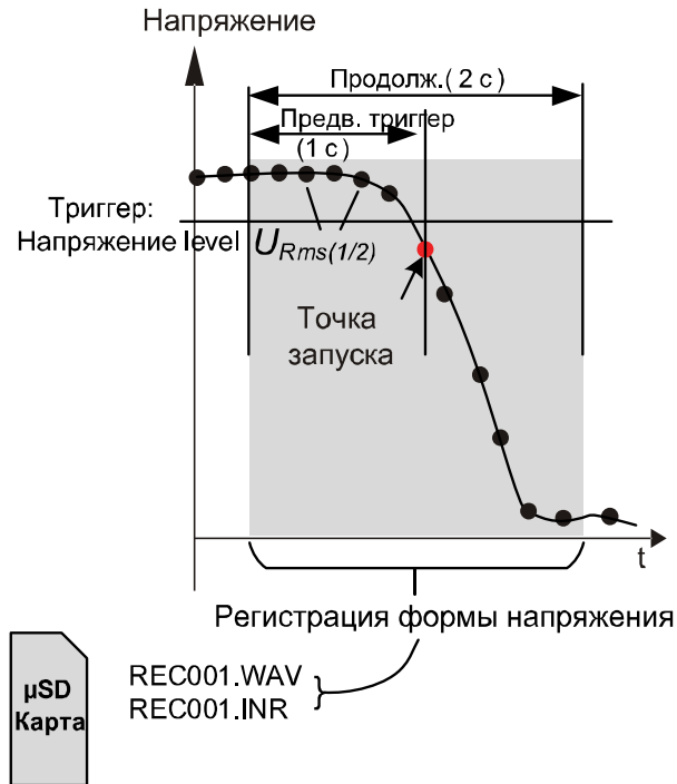
Рисунок 5.22: Формирование триггерного сигнала по уровню напряжения
