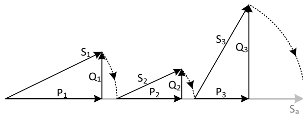
Рисунок 5.5: Арифметическая интерпретация суммарной мощности
