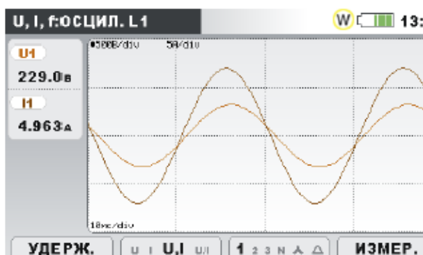
Рисунок 3.5: Форма кривых напряжения и тока (однофазный режим)
