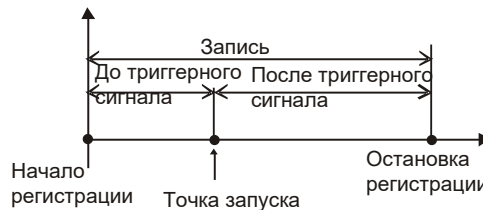
Рисунок 3.1: Триггерные сигналы в регистрации формы напряжения и тока
