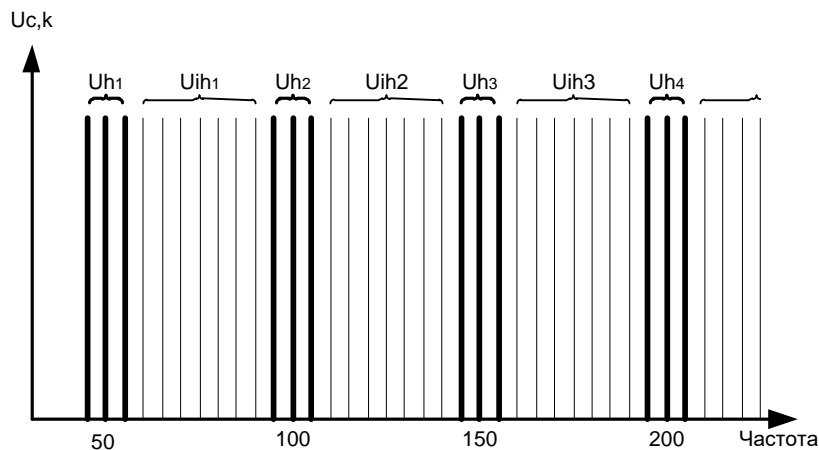
Рисунок 5.9: Иллюстрация подгруппы гармоник/интергармоник для частоты питания 50 Гц
