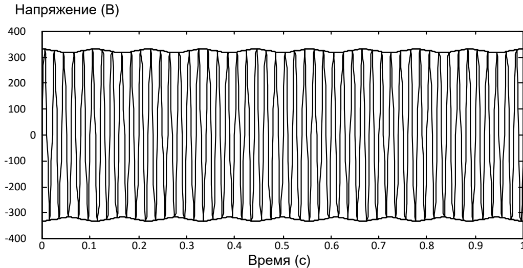
Рисунок 5.10: Колебания напряжения
