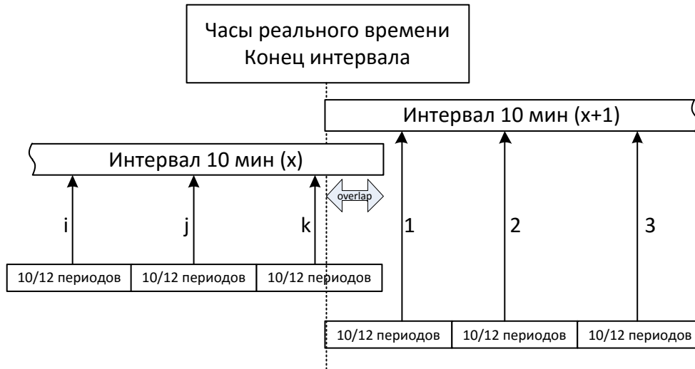
Рисунок 5.16: Синхронизация и объединение интервалов продолжительностью 10/12 периодов
