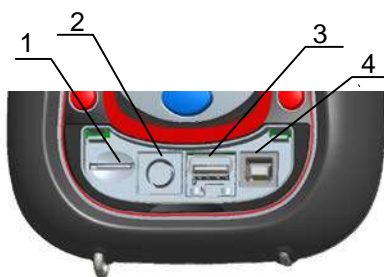
Рисунок 2.2: Боковая панель с разъемами
