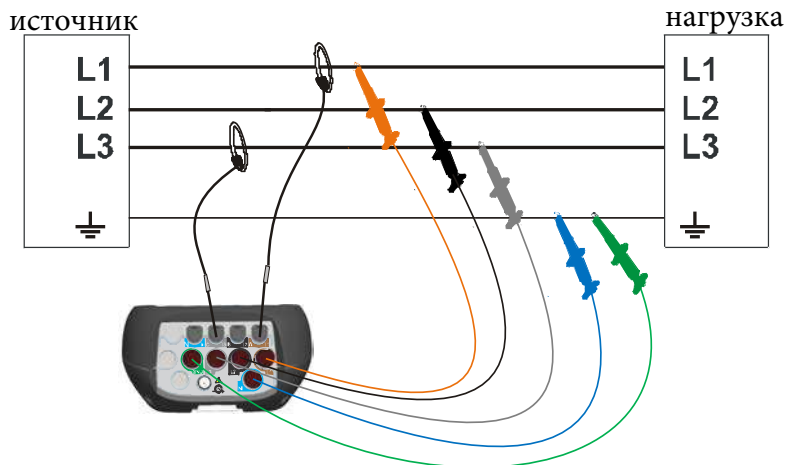
Рисунок 4.7: 3-проводная система « разомкнутый треугольник» (схема Аарона)
