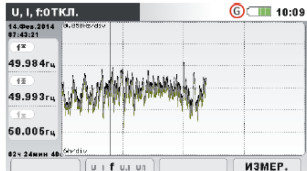
Рисунок 3.12: Отклонения частоты
