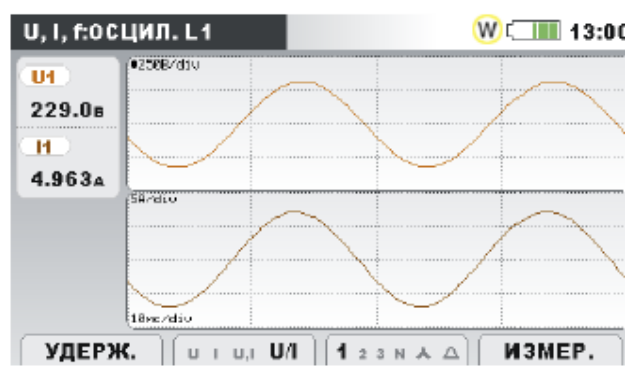
Рисунок 3.6: Форма кривых напряжения и тока (двухфазный режим)
