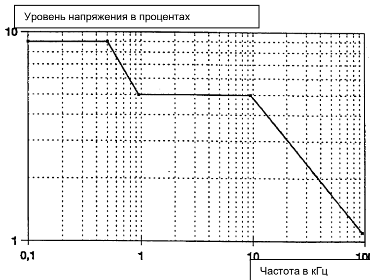
Рисунок 5.1: Предельные уровни сигнальных напряжений, передаваемых по электрическим сетям, согласно стандарту EN50160
