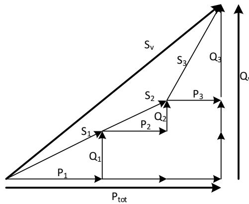
Рисунок 5.4: Векторная интерпретация суммарной мощности
