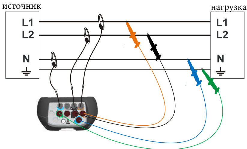
Рисунок 4.11: 2-фазная 4-проводная система
