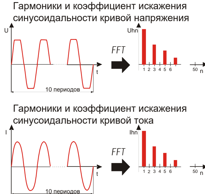
Рисунок 5.8: Гармоники тока и напряжения
