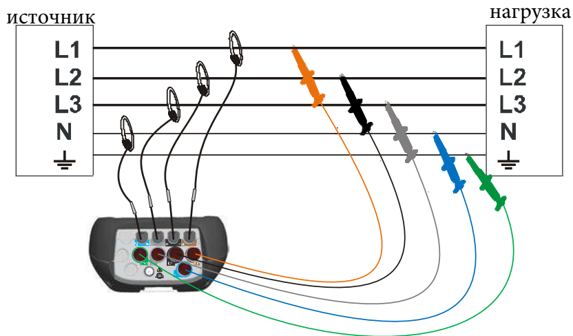
Рисунок 4.3: 3-фазная 4-проводная система
