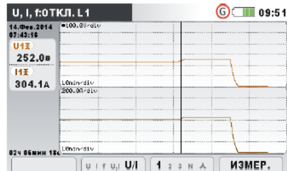
Рисунок 3.10: Отклонения напряжения и тока (двухфазовый режим)
