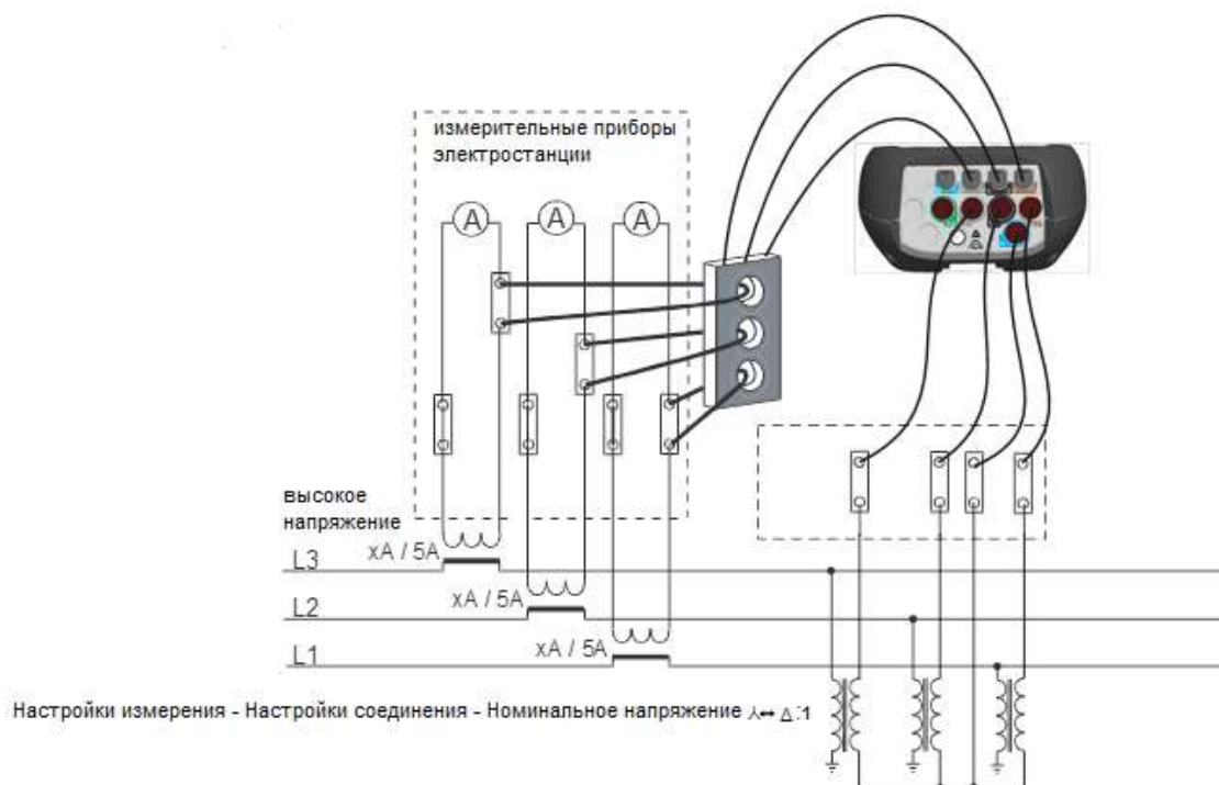
Рисунок 4.16: Подключение прибора к существующим трансформаторам тока в системе среднего напряжения (звезда - звезда)
