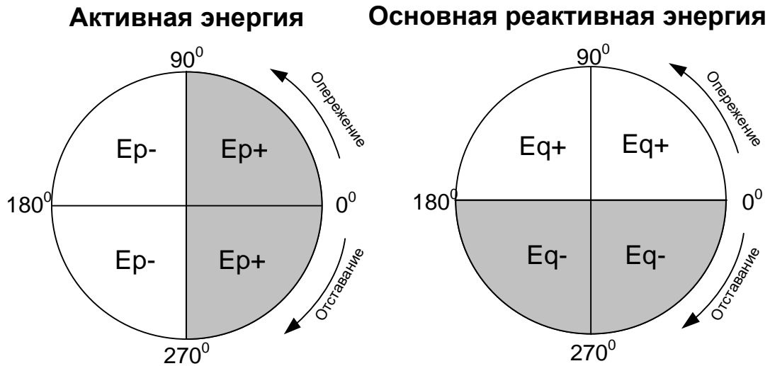
Рисунок 5.6: Соотношения между счетчиками энергии и квадрантами
