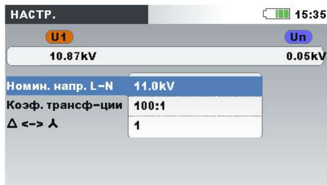
Рисунок 4.12: Ввод коэффициента трансформации для трансформатора 11кВ/110 кВ
