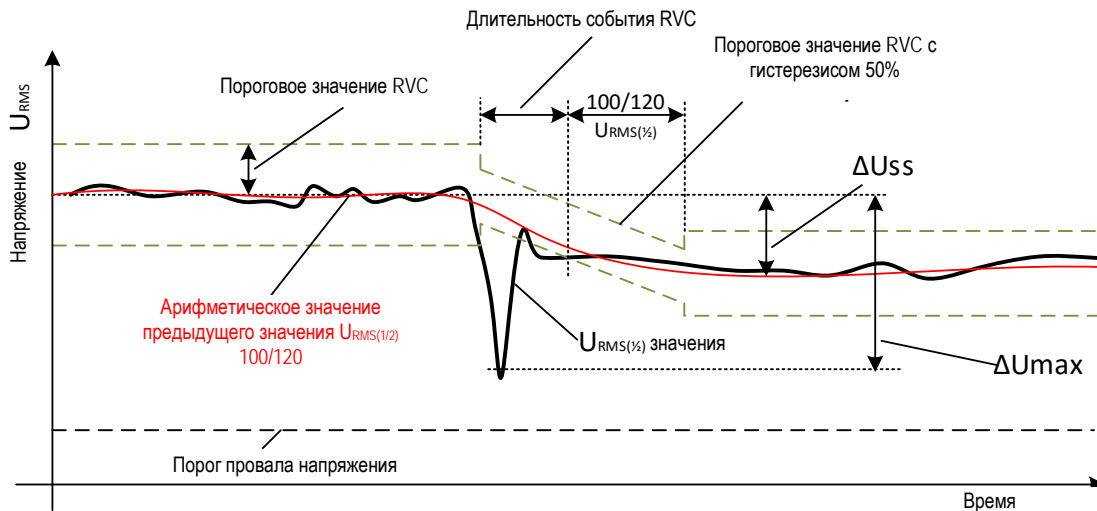
Рисунок 5.15: Описание события RVC
