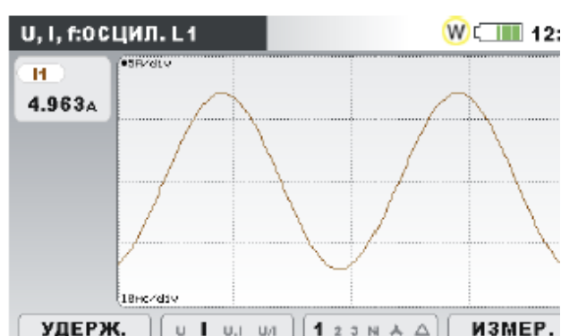
Рисунок 3.4: Только форма кривой тока
