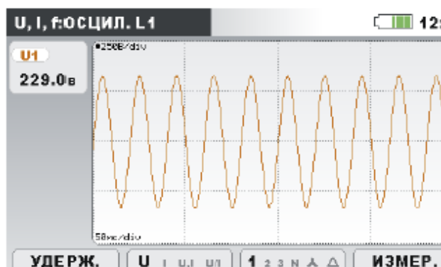
Рисунок 3.3: Только форма кривой напряжения
