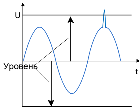
Рисунок 5.28: Триггер обнаружения переходных процессов (уровень)
