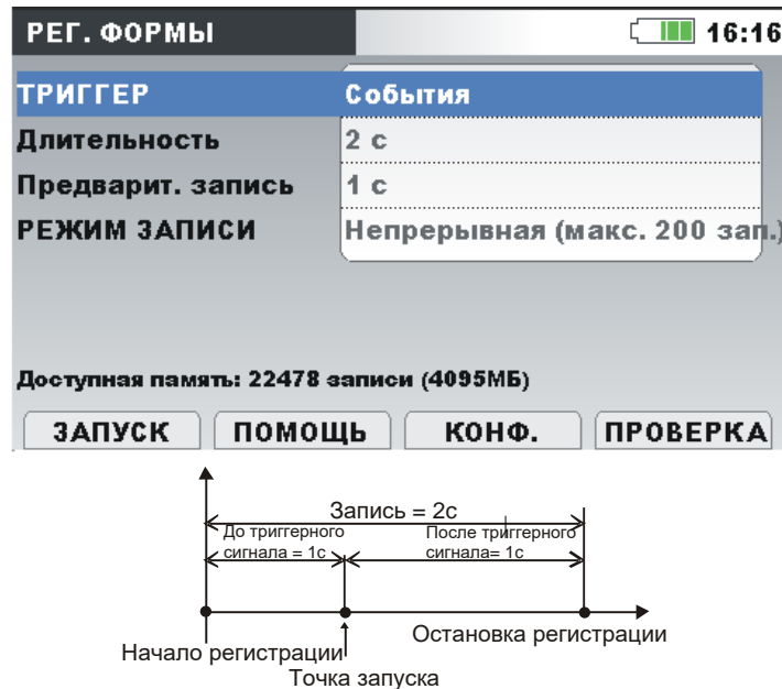
Рисунок 5.20: Формирование триггерного сигнала и период до формирования триггерного сигнала
