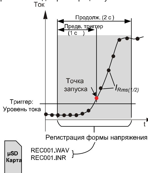
Рисунок 5.23: Формирование триггерного сигнала по уровню тока (пусковой ток)
