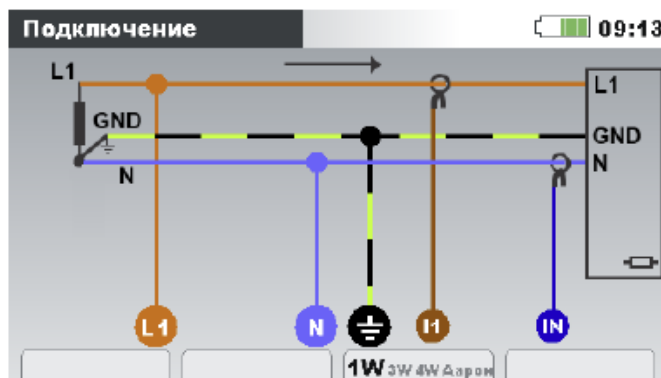
Рисунок 4.8: Выбор 1-фазной 3-проводной системы на приборе
