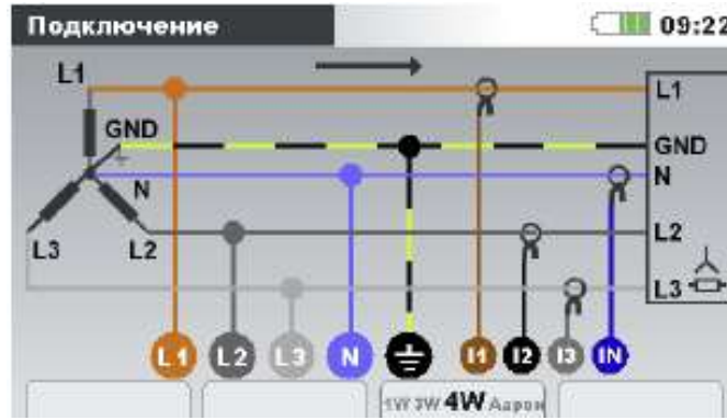
Рисунок 4.2: Выбор 3-фазной 4-проводной системы на приборе
