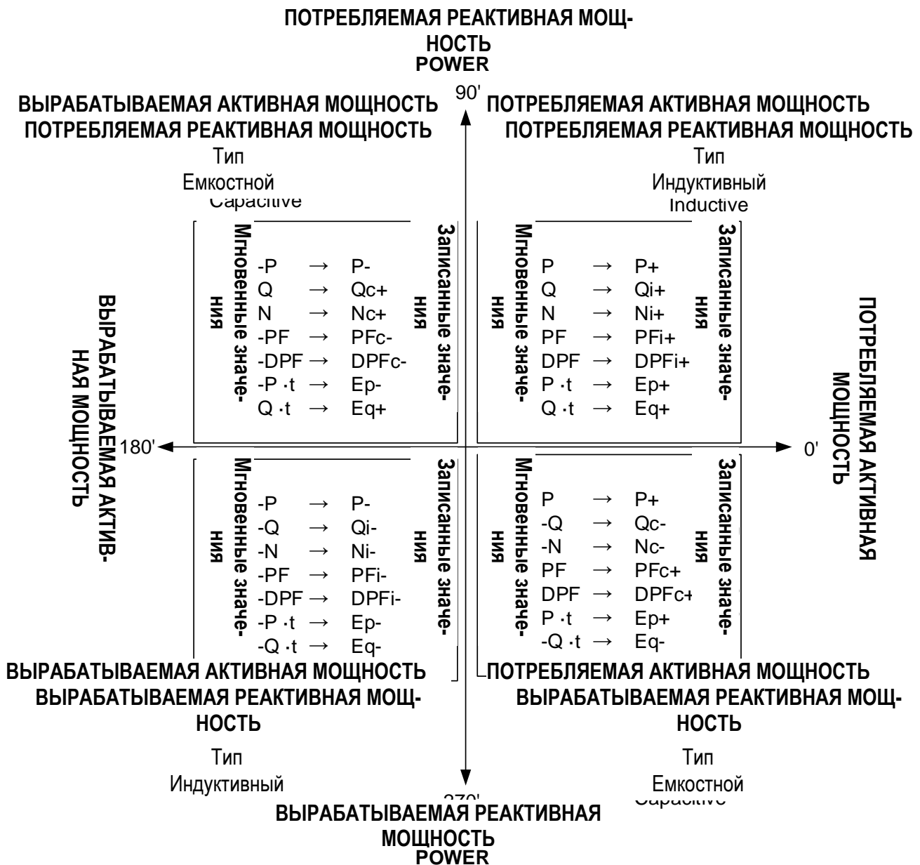
Рисунок 5.18: Фазовая диаграмма/диаграмма полярности потребляемой/генерируемой и индуктивной/емкостной мощности
