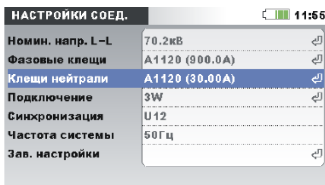
Рисунок 4.21: Настройка автоматически распознаваемых токовых клещей
