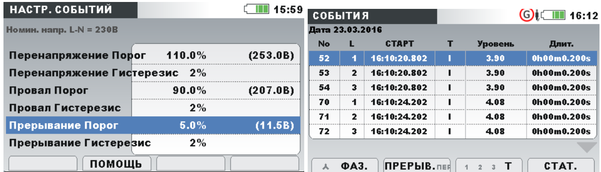
Рисунок 5.14: Экран с данными о прерываниях напряжения
