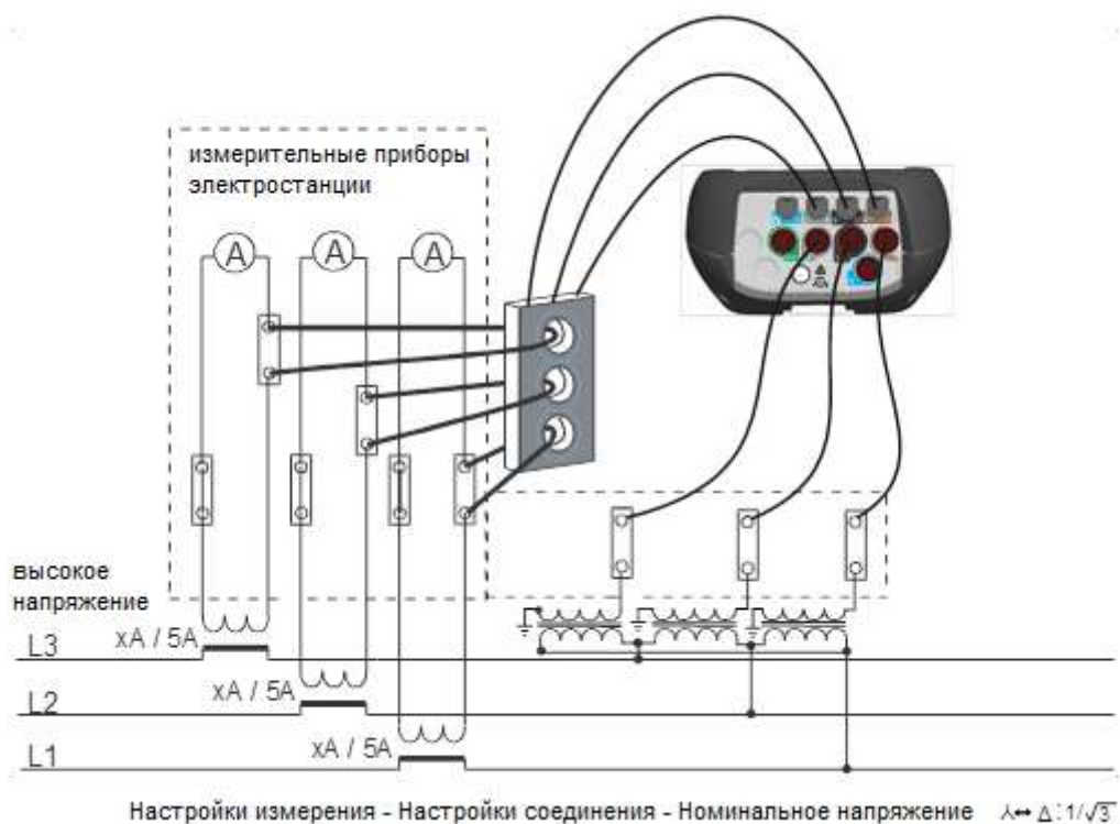
Рисунок 4.15: Подключение прибора к существующим трансформаторам тока в системе среднего напряжения (треугольник - звезда)
