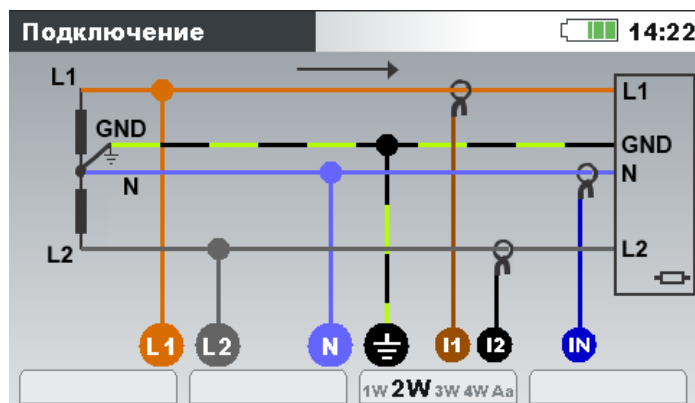
Рисунок 4.10: Выбор 2-фазной 4-проводной системы на приборе
