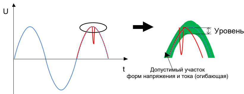
Рисунок 5.27: Обнаружение триггера переходных процессов (огибающая)
