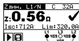
Рисунок 5.32: Примеры результатов измерения импеданса линии
