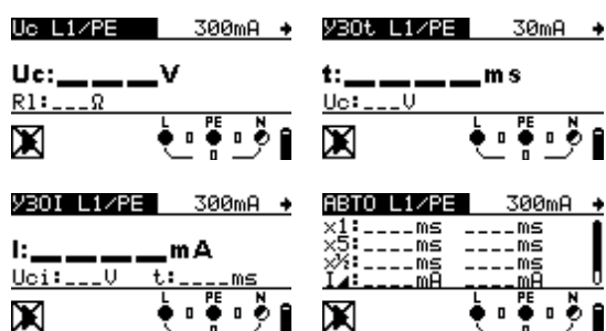
Рисунок 5.19: Тестирование УЗО
