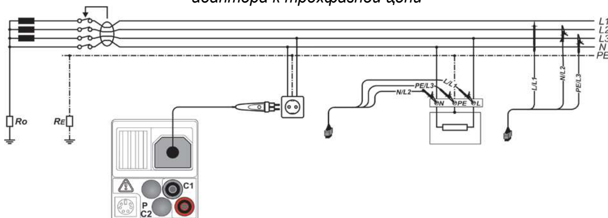
Рисунок 5.3: Подключение штепсельного щупа и 3-х проводного тестового кабеля к однофазной цепи
